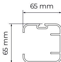
Guías laterales / Lateral guides Guide laterali / Guides latéraux
