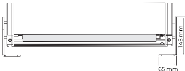
Barra de contrapeso con tracción / Hem bar with traction mechanism Fondale con sistema di trazione / Barre de charge avec système de traction
