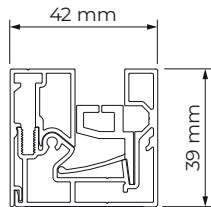
Sección guía superior / Upper guide section Sezione guida superiore / Section top guide
