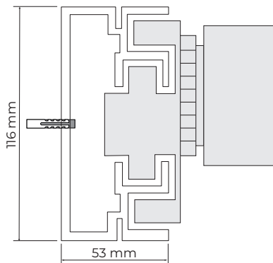
Sección guía lateral / Lateral guide section Sezione guida laterale / Section de guidage latéral
