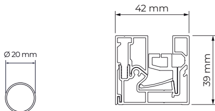
Contrapeso / Hem bar Fondale / Barre de charge
