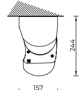
Montaje a techo 90°
