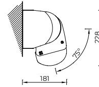
Montaje a pared 75°
